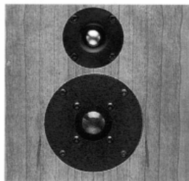
オリジナルのHL5を基本構成として、フロントパツフル最上部に20mmハードドーム・スーパートウィーターを追加。
